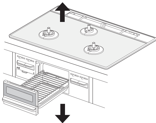
爐頭齒蓋
