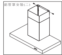
將上鋁管罩與固定片鎖上螺絲固定(如圖三)。
