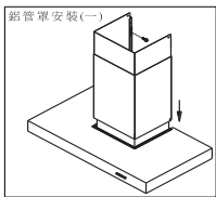
鋁管罩安裝(一) 鋁管罩請依廚櫃設計調整高度固定後，再放至機身凹槽內(如圖二)。
