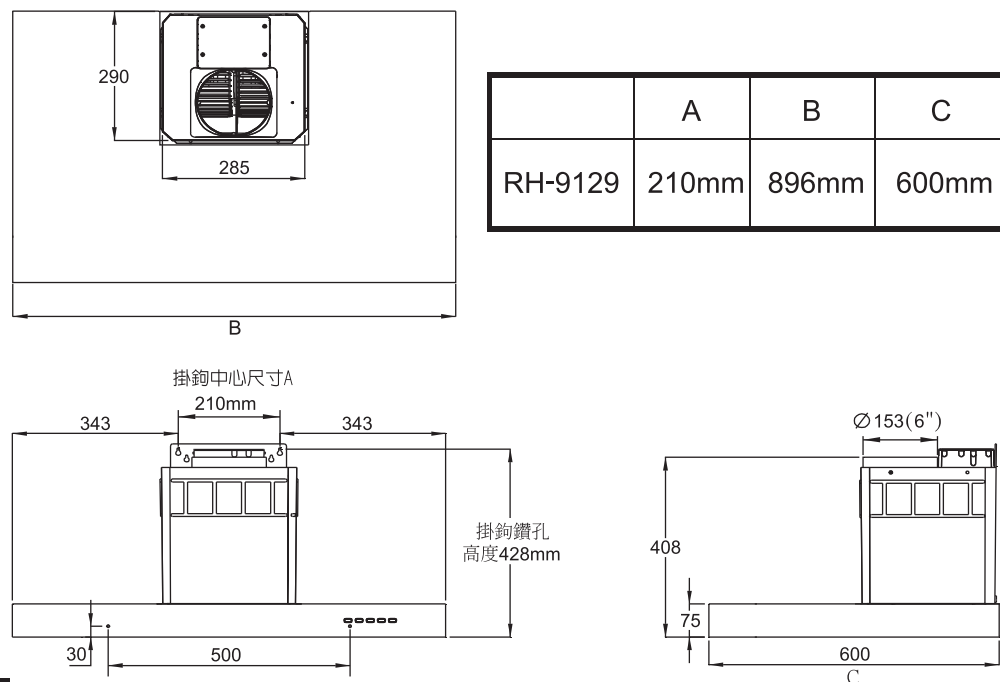
安裝尺寸圖
