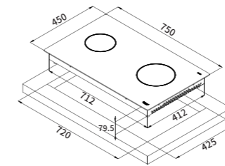
RB-2231HA IH智慧感應雙口爐
