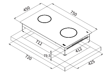
RB-2232HA IH智慧感應雙口爐
