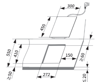
RB-H1180 IH智慧感應單口爐
