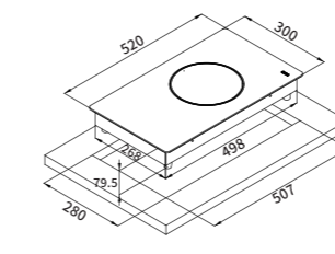
RB-1132H IH智慧感應單口爐
