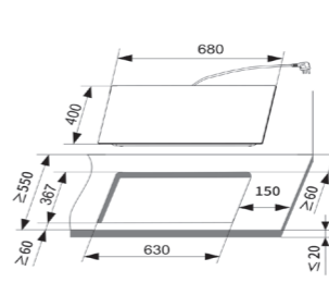
RB-H2280A IH智慧感應單口爐
