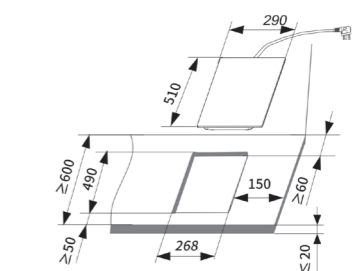
RB-H2180 IH智慧感應雙口爐(縱向)
